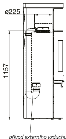
koaxiální zapojení 905SV
