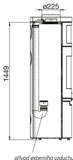
koaxiální zapojení 905BV
