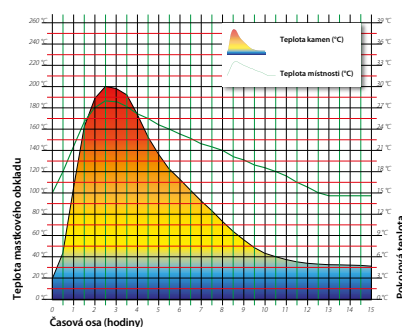
Test akumulace Pecan Eco M (použité palivo 8,5 kg olšového dřeva s obsahem vlhkosti do 16 %)
