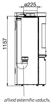
koaxiální zapojení 905V
