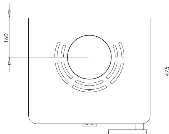
Vzdálenost kamen od hořlavých materiálů:
