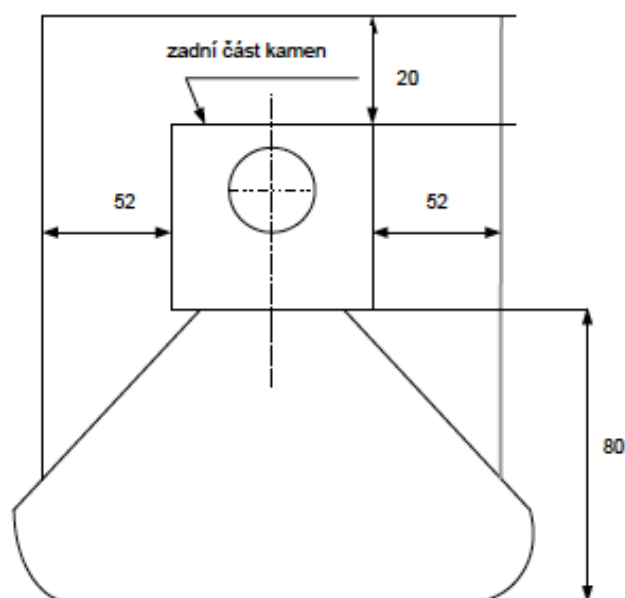
Vzdálenost kamen od hořlavých materiálů:
