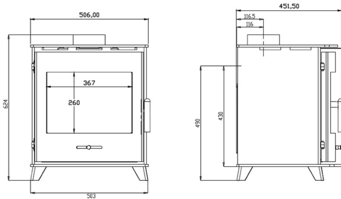
Technický výkres hede 6:
