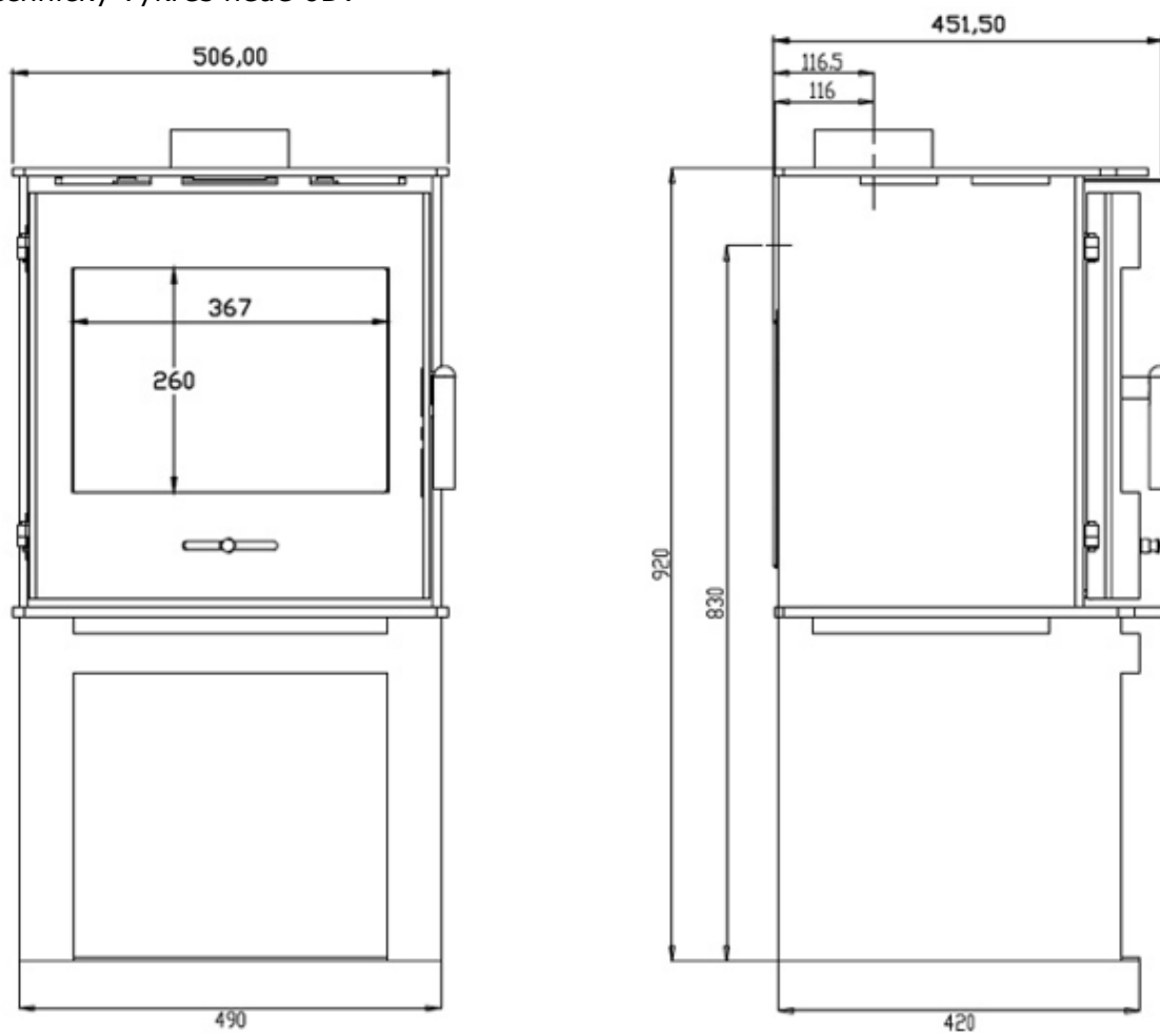
Technický výkres hede 6D:
