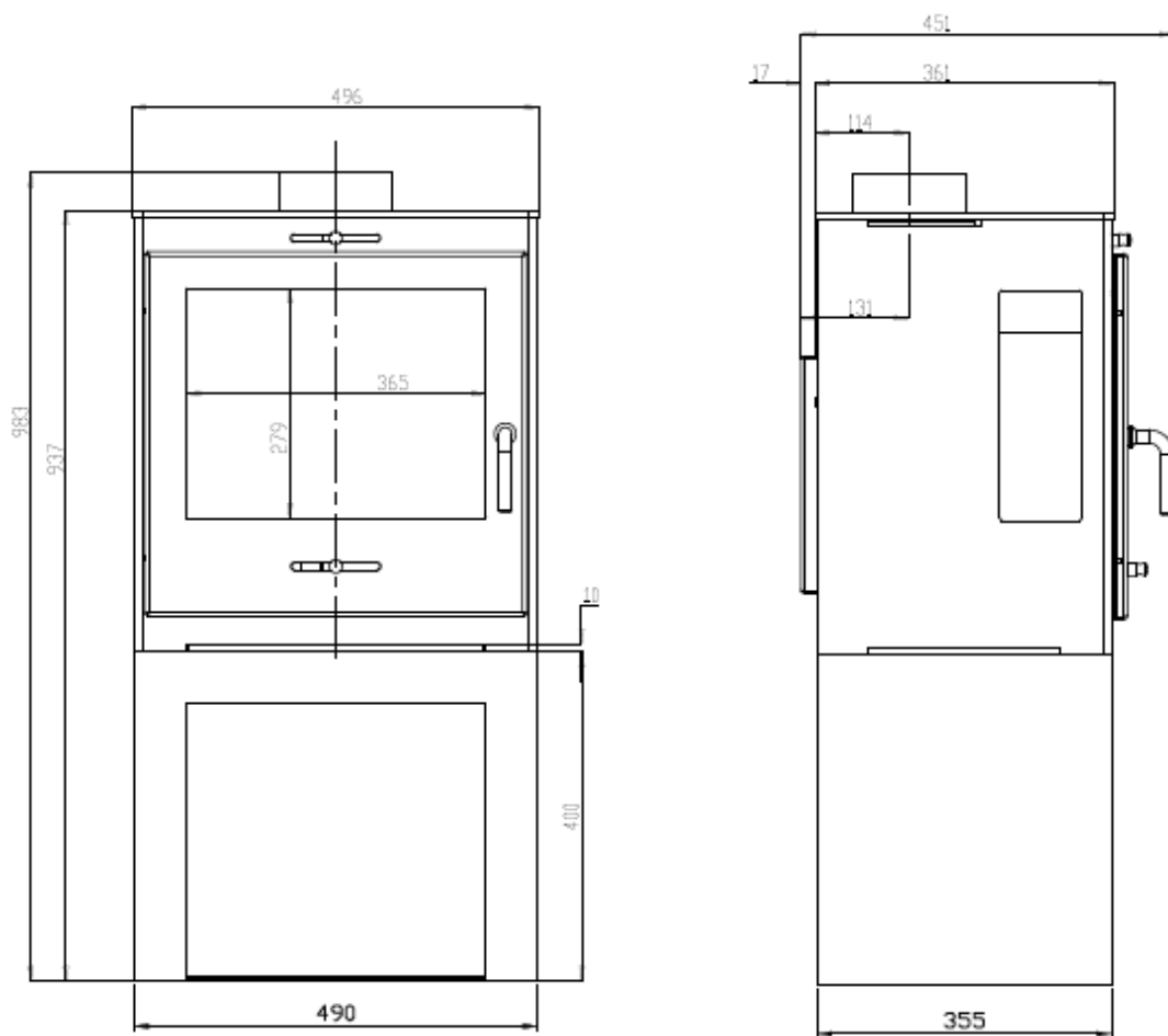
Technický výkres hede 2D Panorama:
