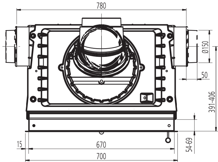
VIDA 68 F Draufsicht / M1:10
