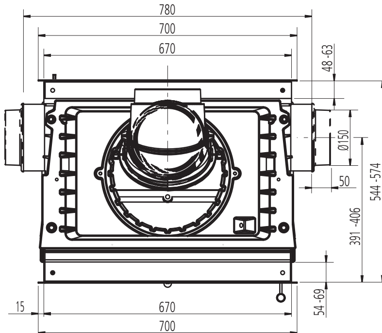
VIDA 68 DS Draufsicht / M1:10
