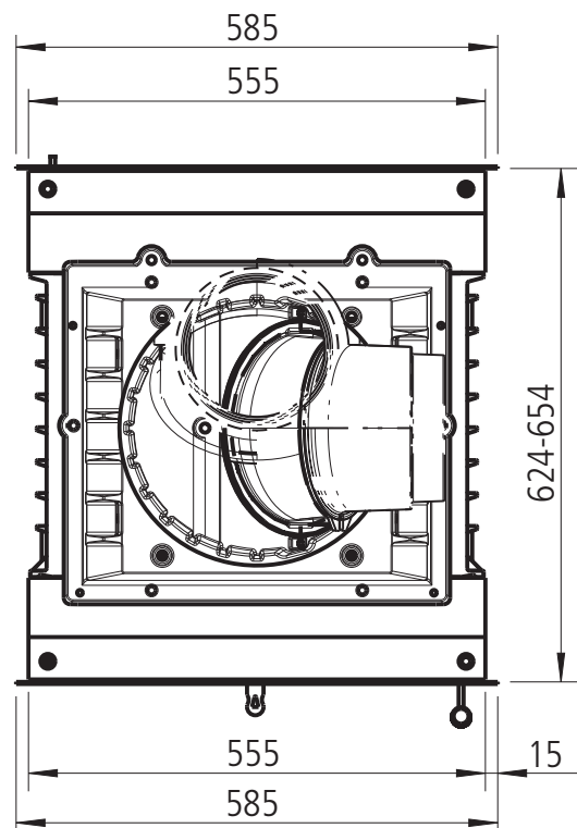
VIDA 55 DS Draufsicht / M1:10
